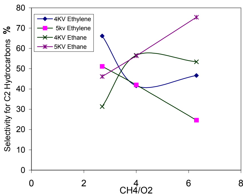
شکل ۹ - تاثیر نسبت خوراک بر گزینش‌پذیری به اتان و اتیلن در دمای ۳۰۰ درجه سانتی‌گراد
