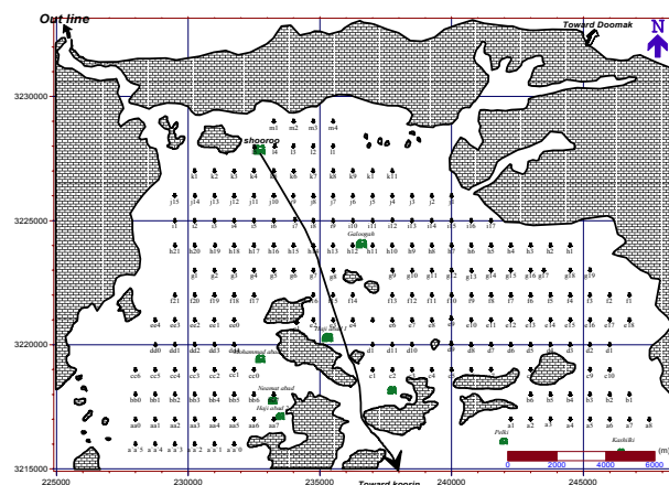
شکل ۱- محدوده دشت شورو و سونداژهای برداشت شده در آن [۴]
