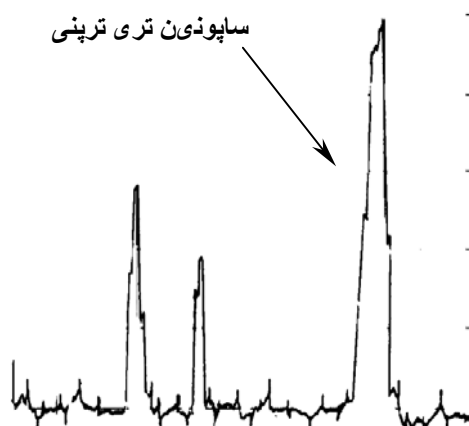
شکل ۲- کروماتوگرام مربوط به ساپونین در نمونه کنترل
