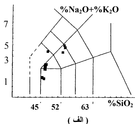
شکل ۳- الف) دیاگرام TAS برای طبقه‌بندی سنگ‌های ولکانیک (طبق توصیه‌های IUGS به نقل از لومتر ۱۹۸۹ براساس لوپاس و دیگران ۱۹۸۶ ب) زیرتقسیمات بعدی تراکی بازالت و تراکی آندزیت (لومتر ۱۹۸۹ با اقتباس از شلی ۱۹۹۱)
