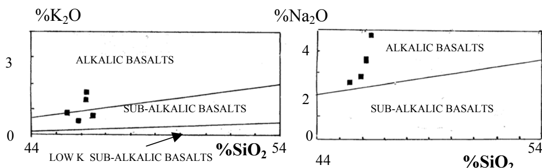
شکل ۵- طبقه‌بندی بازالت‌های آکالیک و ساب آکالیک (نقل از میدل موسست ۱۹۷۵، اقتباس از ویلسون ۱۹۹۷)
