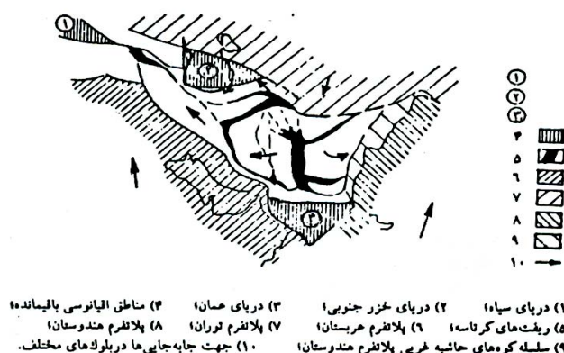
شکل ۲۳- شکلی از کلیه ریفتهای کرتاسه در محدوده صفحه ایران - افغانستان ( اشتامپلی ۱۹۷۸ برگرفته از کتاب زمین‌شناسی ایران علی درویش زاده ۱۳۸۰) امتداد این ریفتهای در جهت خطوط غیر ممتد ظاهراً از منطقه مورد مطالعه می‌گذرد.
