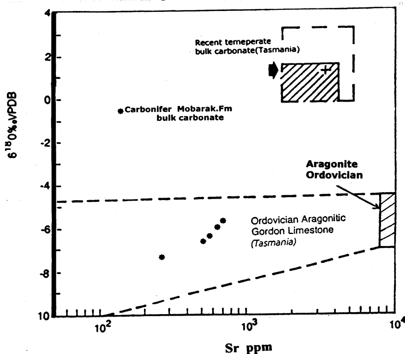
شکل ۱۲- تغییرات ایزوتوپ اکسیژن در مقابل Sr. در این نمودار نمونه‌های کربناته سازند مبارک درون محدوده آهک‌های آراگونیتی اردوئیسین (رائو، ۱۹۹۰) واقع شده است که این به دلیل مشابهت کانی شناسی بین این دو حوضه می‌باشد.
