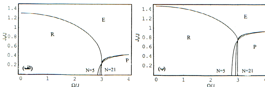
شکل ۲. دیاگرام‌های فاز در صفحه (\Omega_s/J, J_s/J) برای فیلم‌هایی با یک لایه سطحی ( N_s=1 ) که در آن R مربوط به فاز کاهش یافته (T_c(\text{film}) < T_c(\text{bulk})) و E مربوط به فاز افزایش یافته (T_c(\text{film}) > T_c(\text{bulk})) و P فاز پارالکترونیک است. (الف) \Omega_s/J=1 (ب) \Omega_s/J=2
