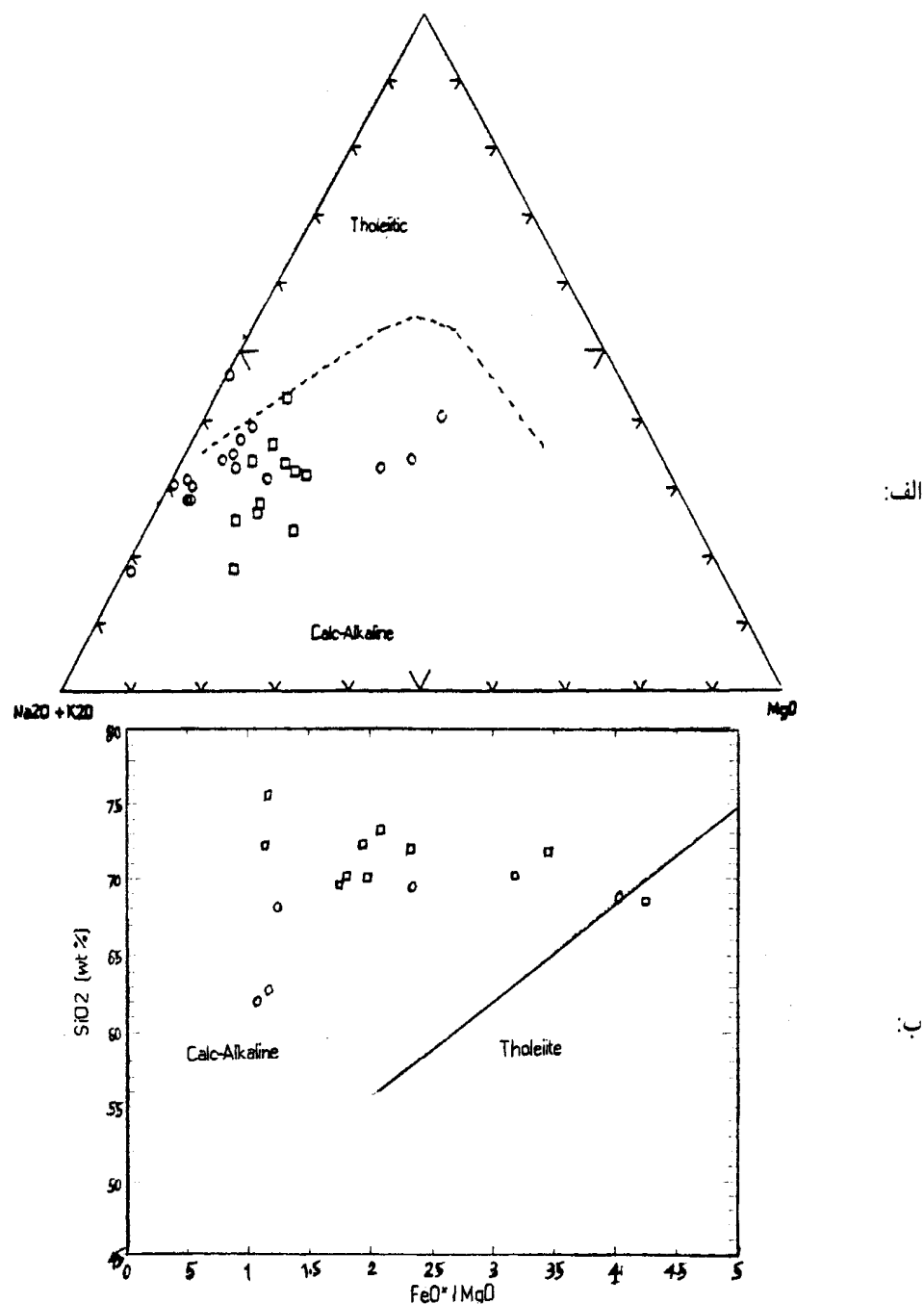
شکل ۷: الف: نمودار ایزوین و بارآگار (۱۹۷۱) و (ب): میاشیرو (۱۹۷۴) که سری‌های کالکوالکالن و تولیت را از هم جدا می‌کند. نمونه‌های منطقه مورد مطالعه در هر دو نمودار خصوصیات کالکوالکالن را نشان می‌دهند.
