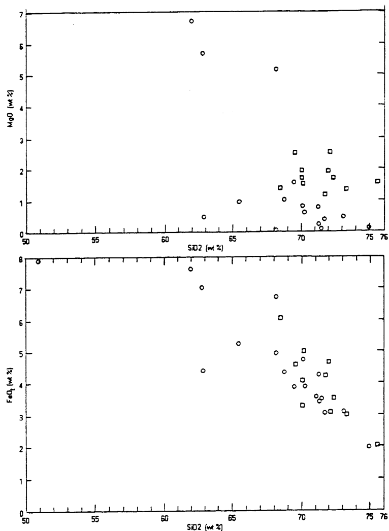
شکل ۴: نمودار تغییرات MgO و FeO در مقابل \text{SiO}_2
