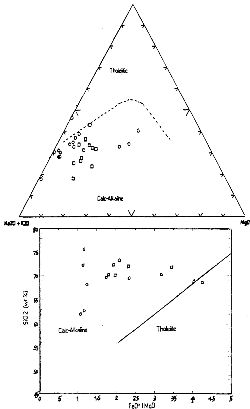
شکل ۷: الف: نمودار ایزوین و بارآگار (۱۹۷۱) و (ب): میاشیرو (۱۹۷۴) که سری‌های کالکوالکالن و تولیت را از هم جدا می‌کند. نمونه‌های منطقه مورد مطالعه در هر دو نمودار خصوصیات کالکوالکالن را نشان می‌دهند.
