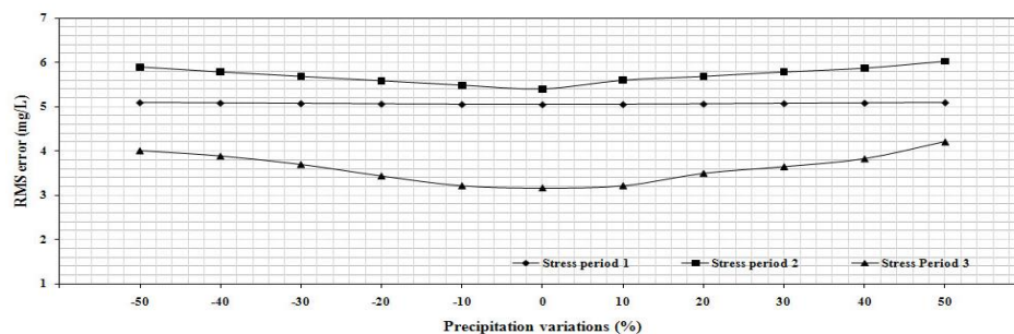
شکل ۱۲. حساسیت مدل انتقال محدوده بررسی شده به تغییرات میزان نفوذ نیترات از طریق بارش
