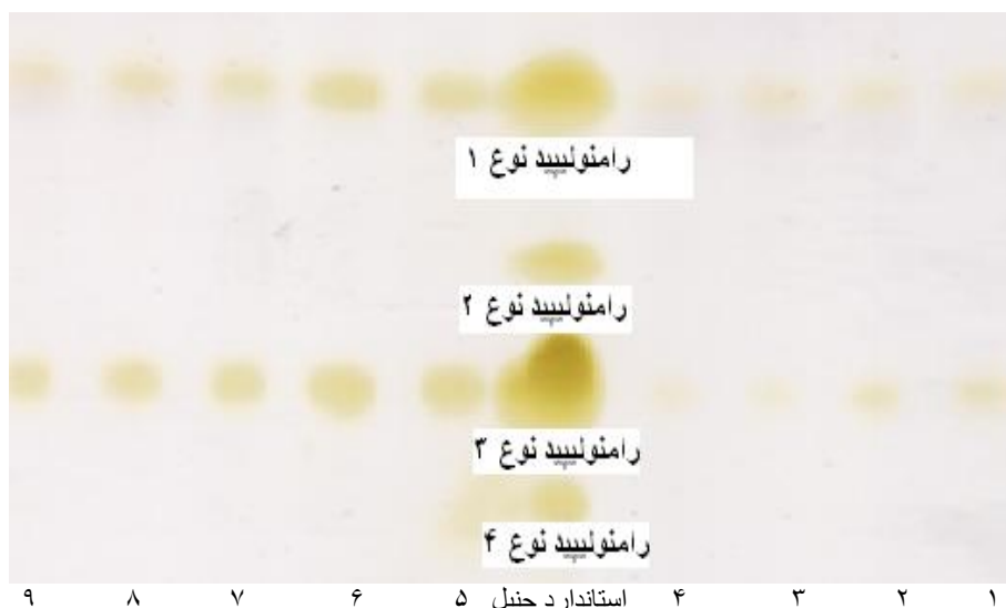
شکل ۴. نتایج کروماتوگرافی از محصول به‌دست آمده از ۹ آزمایش طراحی شده به‌وسیله تاگوچی با استفاده از لایه چهار لکه وسط به‌عنوان شاهد از استاندارد جنیل به‌دست آمده است
