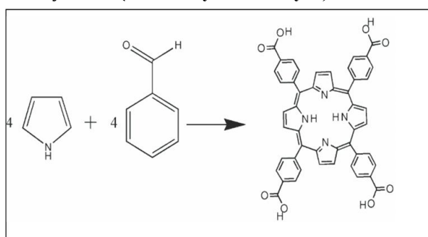
شکل ۲. واکنش شیمیایی سنتر پورفیرین
