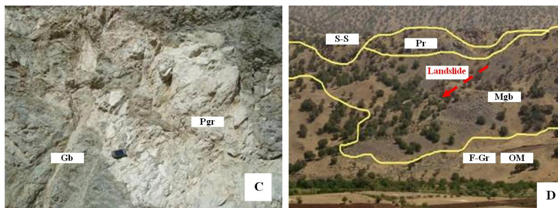
شکل ۲. (C) نفوذ دایک‌های فلسیک پلاژیوگرانیتی (Pgr) در گابروها و میکروگابروها (F-Gr) در گابروها، (D) راندگی اسلیت‌های سنندج سیرجان (S-S) روی پریدوتیت (Pr) و میکروگابرو (مجموعه افیولیتی) و کل مجموعه روی واحد اولیگومیوسن (OM)
