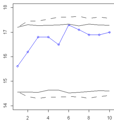
شکل ۵. بازه‌های پیش‌گویی ۱ گام آینده میانگین دمای هوای
