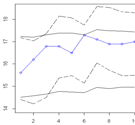
شکل ۶. بازه‌ی پیش‌گویی بوت‌استرپ ۱۰ مشاهده
