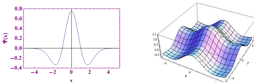
شکل ۱. شکل ۲ بعدی و ۳ بعدی موجک کلاه مکزیکی، که به‌ازای N=2 و یا N=3 به‌دست می‌آید
