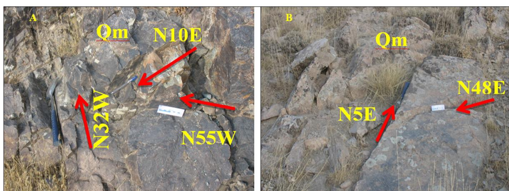
شکل ۴. ساختارهای زمین‌شناسی مشاهده شده در منطقه ذاکر
