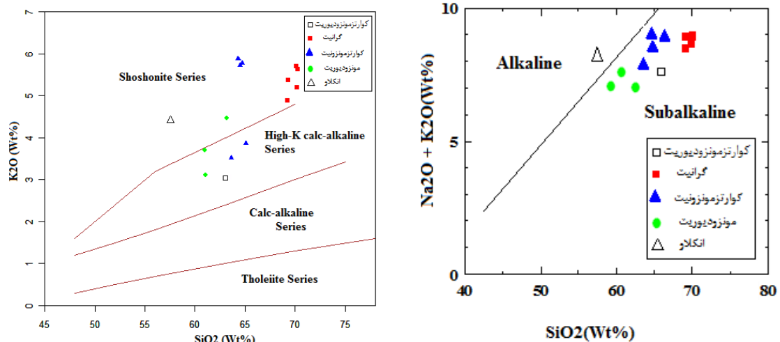
شکل ۱۰. نمودار آلكالی در برابر سیلیس [۱۵]
