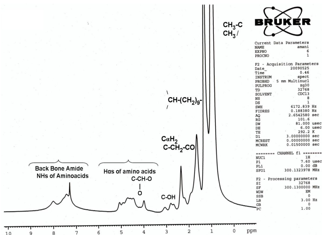
شکل ۴. طیف H NMR سورفکتین تولید شده از باکتری باسیلوس سابیتیلیس ۰۱۱۰ NLIM تحت شرایط بهینه بیوراکتور (۳۷ °C و ۳۰۰ rpm و ۵ / ۱ vvm)
