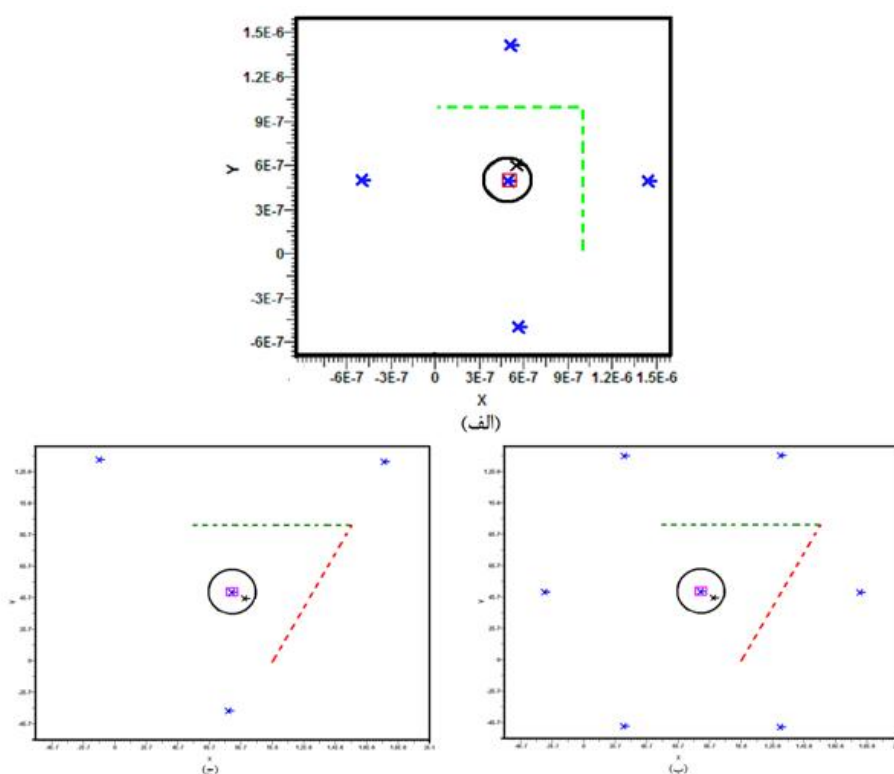
شکل ۳. چیدمان میله ها (مرزها)، چندقطبی ها، بسط های بسط و مرز تناوبی فرضی خط چین الف) ساختار مربعی، ب) ساختار مثلثی، ج) ساختار لانه زنبوری
