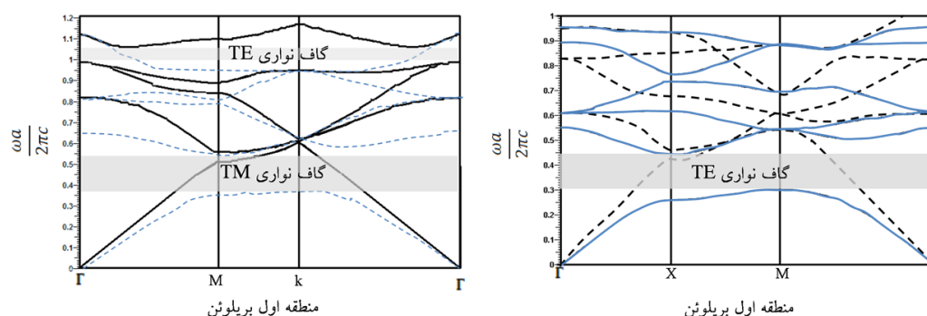
شکل ۶. راست) ساختار نواری شبکه مربعی متشکل از میله های دی الکتریک r=0.18a با گذردهی 11/56 در هوا قطبش خط TE، خط چین TM، چپ) ساختار نواری شبکه مثلثی متشکل از میله های دی الکتریک r=0.15a با ضریب گذردهی 8/41 در هوا قطبش خط TE، خط چین TM
