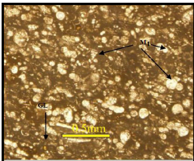
شکل ۱۰. افزایش درصد مورفوتایپ نوع ۱ (M1) و کاهش گلوکونیت (GL) و فسفات (PH) و ضعیف شدن بافت در مرزهای سکاسی در نمونه G12
