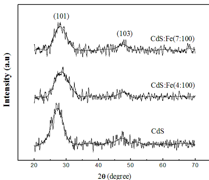
شکل ۲. طرح پراش اشعه ایکس نانوذرات CdS آلاییده و غیرآلاییده. ([TG]= ۰/۰۹ M)
