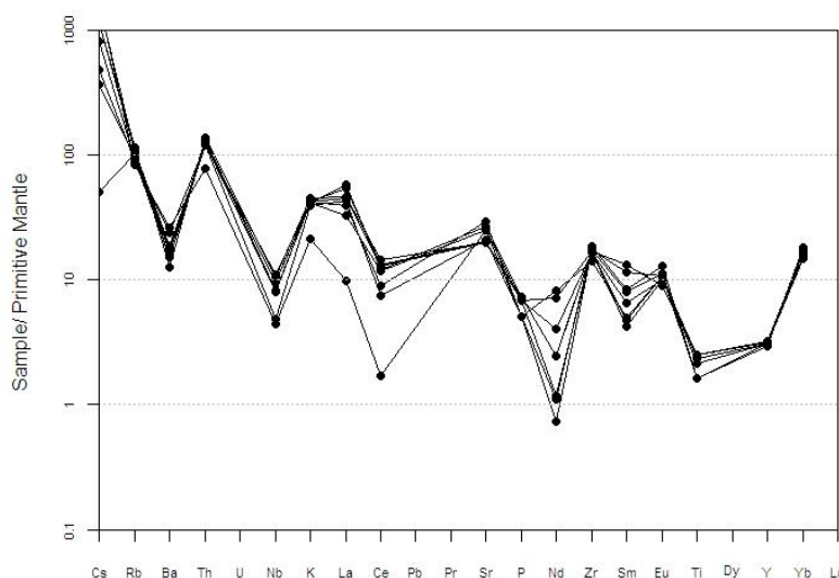
شکل ۶. نمودار چند عنصری به نهار شده نسبت به گوشته اولیه [۲۲]، ناهنجاری مثبت عناصر Sr و Eu را می‌توان به عدم جدایش و ته نشست ثقیل پلاژیوکلازها نسبت داد. در ضمن الگوهای به نسبت یک‌نواخت نمونه‌ها نشان می‌دهد که تفاوت‌های ژئوشیمیایی کمی بین سنگ‌های بررسی شده وجود دارد
