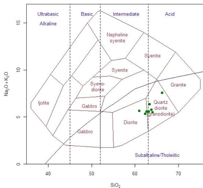
شکل ۲. موقعیت نمونه‌های بررسی شده در نمودار مجموع آلکالن (TAS) در برابر \text{SiO}_2 [۱۷]. اغلب سنگ‌ها در محدوده ترکیبی کوچکی بین دیوریت و کوارتز دیوریت قرار گرفته‌اند
