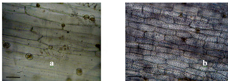
شکل ۶. سلول‌های اپیدرمی ساقه در (a) اوتریکولاریا استرالیس و (b) اوتریکولاریا مینور به کمک میکروسکوپ نوری با بزرگنمایی ۴۰
