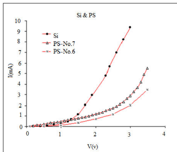
شکل ۷. نمایش اثر خوردگی بر رسانندگی نمونه‌ها. مشاهده می‌شود که پس از تخلخل رسانندگی نمونه‌ها کم می‌شود. این نتیجه با آنچه در شکل ۶ آمده است در تطابق است. هرچه گاه انرژی نمونه بیش‌تر باشد رسانندگی آن کمتر است.
