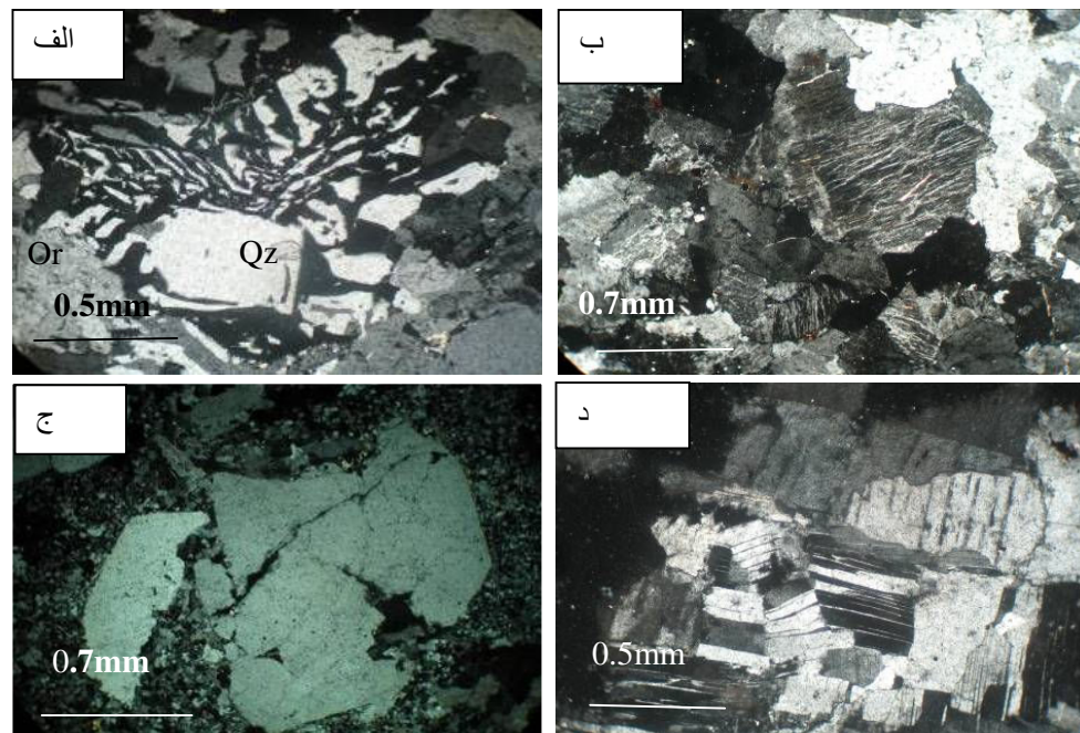
شکل ۲. الف) بافت‌های گرانوفیری در گرانیت زیریگان. ب) پرتیت رشته‌ای. ج) شکستگی بلور کوارتز (ساب گرین) در اثر تنش تکتونیکی در گرانیت چاه چوله د) شکستگی پلاژیوکلاز در اثر تنش و تجمع موزاییکی
