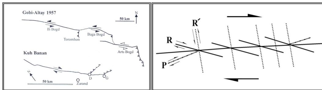
شکل ۱۸. تشکیل شکستگی‌های R و R'
