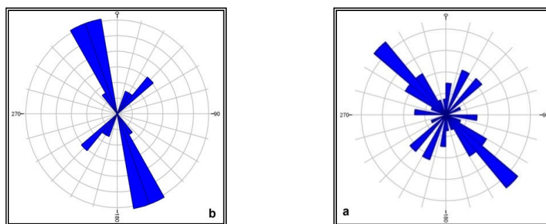
شکل ۱۰. دیاگرام گل‌سرخ‌گی‌ها (a) و درزه‌های (b) زون گسل اسلام‌آباد
