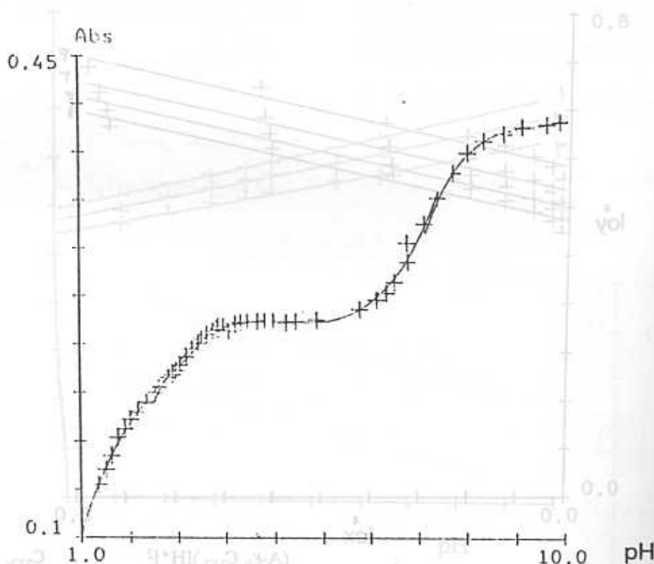
شکل ۱: تغییرات جذب بر حسب pH برای کمپلکسهای VO_2^+ - گلوتامیک اسید، در 25^\circ C و در طول موج ۲۶۵ نانومتر.
