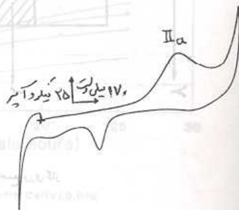
شکل ۲: ولتاموگرام چرخه‌ای محلول 5M H_2SO_4 و در سطح الکترود Pt. محدوده پتانسیل ۱۰۵ تا ۱۵۵۰ میلی‌ولت. سرعت جاروب 30mv/sec.
