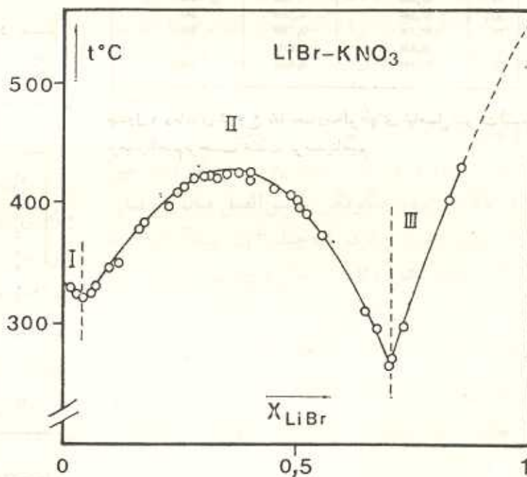
شکل ۳ نمودار تغییر دمای شروع به انجاماد بر حسب غلظت در سیستم نیترات پتاسیم- برمید لیتیم
