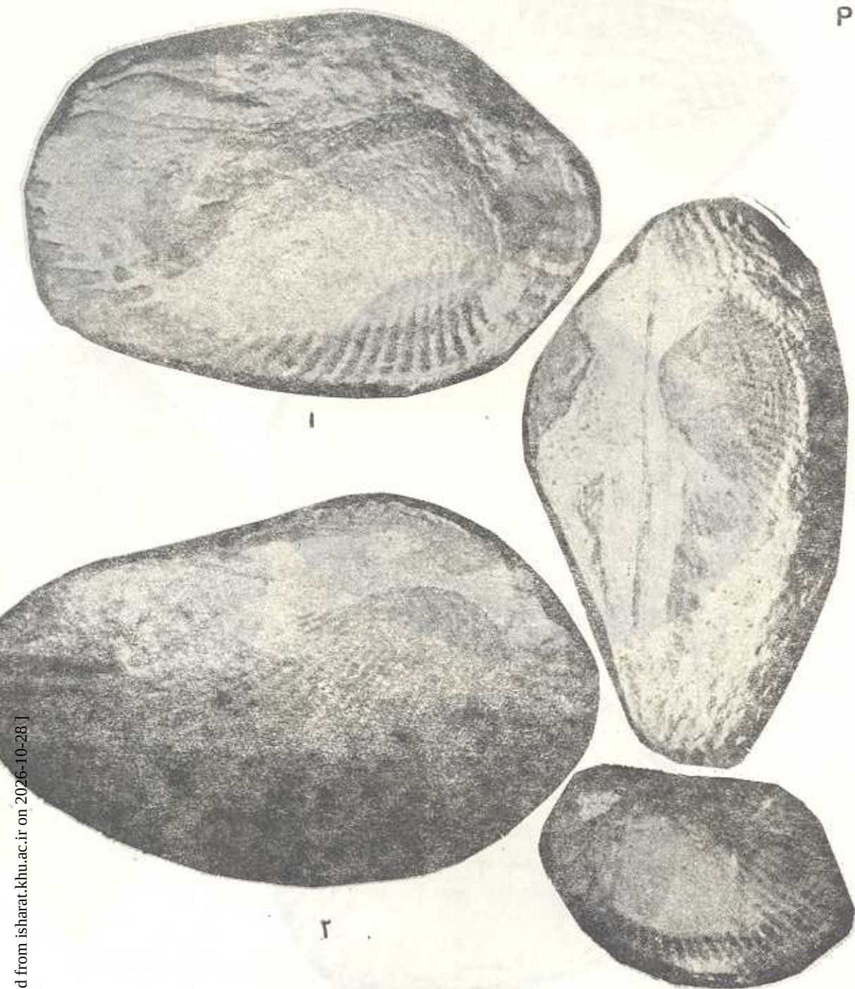
شکل ۱ و ۲ : منظره سطح پستی کفهای چپ از گونه Anadara (Gr.) Pectinata Br. ۳ : از نیم رخ : طرز قرار گرفتن کروشها و سطح کاردینال را نشان می دهد. ۴ : طرز قرار گرفتن دندها و حدفصل آنها در روی کف راست.
