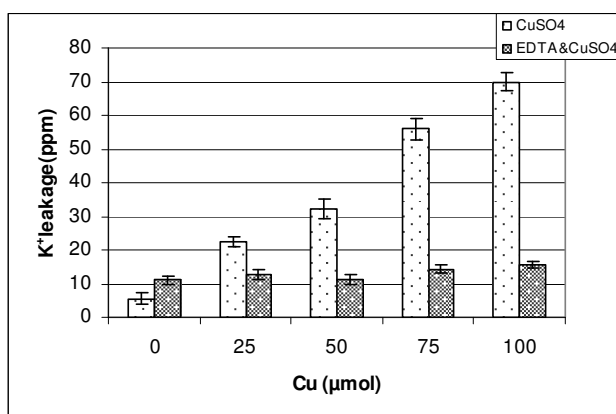
نمودار ۳. اثر تراکم‌های مختلف مس و (مس + EDTA) بر نشت یون پتاسیم به محیط کشت در گیاه ذرت بارهای عمودی مس و مس + EDTA گویای SE \pm است.
