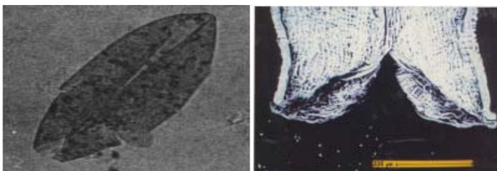
شکل ۱۶. تصویر SEM از دهانه دو عضو کنودونت که از پهلوی به هم چسبیده‌اند.
