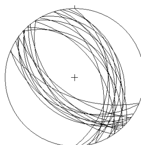
شکل ۸. الف) نمودار برگوارگی‌های نسل اول که دارای راستای شمال شمال باختر جنوب جنوب هستند ب) برگوارگی‌های نسل دوم در یک جین از نوع کینک در سنگ‌های سیلورین، خاور رشم. نگاه به جنوب باختر اندازه قلم داخل کادر: ۸ س.م
