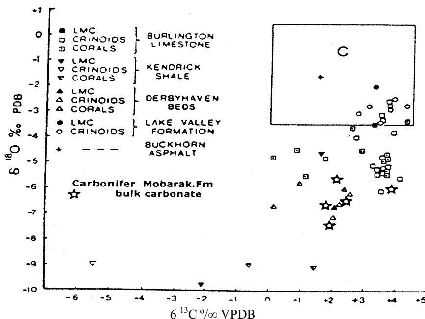
شکل ۱۱- تغییرات ایزوتوپ اکسیژن ۱۸ و ایزوتوپ کربن ۱۳ در نمونه‌های کل کربناته سازند مبارک و مقایسه آن با محدوده فسیلهای آلتره نشده آراگونیت و کلسیت کم منیزیم. محدوده C محدوده فسیلی کربونیفر برای آن دسته از ترکیباتی که در حال تعادل ایزوتوپی با آب دریا میباشند (دیکسون و کلمن ۱۹۸۰). نمونه‌های کربناته سازند مبارک در نزدیک محدوده ارائه شده توسط دیکسون (۱۹۸۰) و مربوط به توالیهای دریی هاون قرار میگیرند. مقادیر ایزوتوپ کربن سازند مبارک در حد نمونه‌های محدوده C است، ولی ایزوتوپ اکسیژن ۱۸ بعلاوه تأثیر عمده دیانژن متتوریکی مقادیر سبکتری را نشان می‌دهد.
