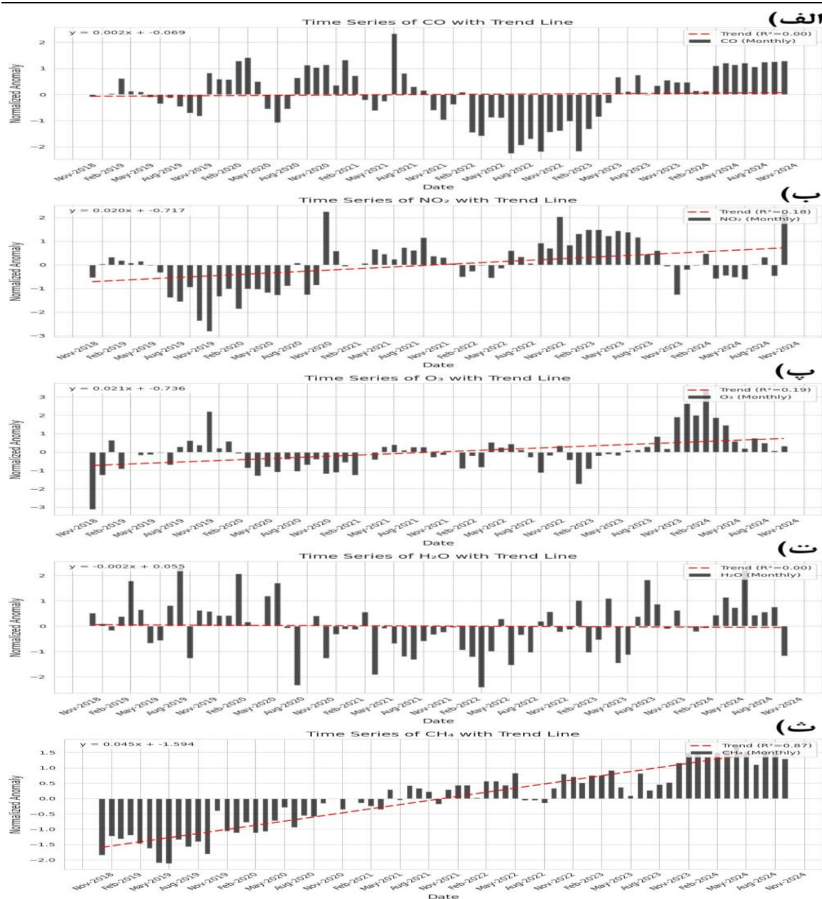
شکل ۳. نمودارهای سری زمانی گازهای گلخانه‌ای (مونوکسیدکربن، دی‌اکسید نیتروژن، ازن، بخار آب و متان) در طی دوره ۲۰۲۴-۲۰۱۹ براساس نتایج حاصل از تحلیل مؤلفه‌های اصلی (PCA)، اکثر متغیرهای گازهای گلخانه‌ای از الگویی با پراکنش یکنواخت و روند افزایشی در طول ماه‌های سال‌های مورد مطالعه پیروی می‌کنند. پارامترهای متان، ازن و دی‌اکسید نیتروژن بیش‌ترین سهم را در تغییرات واریانس کل در تجزیه و تحلیل آماری به خود اختصاص داده‌اند. نتایج تحلیل مؤلفه‌های اصلی نشان داد که حدود ۷۱/۲۷ درصد از تغییرات کل، با دو مؤلفه‌ی (PCA 1 ) و (PCA 2 ) قابل توجیه است. همچنین، تغییرات پارامترهای گازهای گلخانه‌ای در طول ماه‌های سال‌های متوالی، بر اساس یافته‌ها و خروجی PCA، در قالب گروه‌های مختلف ارائه شد. گروه الف: در ماه‌های (ژانویه، فوریه، جولای، آگوست، آوریل، مارس و نوامبر) سال ۲۰۱۹، ماه‌های (سپتامبر و اکتبر) ۲۰۲۰ و ماه‌های (آوریل، فوریه، دسامبر، ژانویه و ژوئن) ۲۰۲۱ کم‌ترین مقادیر غلظت گازهای گلخانه‌ای در کل ستون جو، از سطح زمین تا بالای جو مشاهده شد. در این گروه یک ارتباط تقریباً منظم در رفتار غلظت گازها در طی ماه‌های مذکور دیده شد یعنی با توجه به این که هر چه از ماه‌های سرد به سمت ماه‌های گرم (تقریباً اواخر زمستان تا اوایل تابستان)، غلظت برخی از گازهای گلخانه‌ای روندی اندک افزایشی
