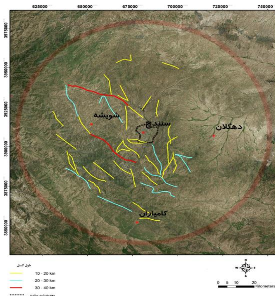
شکل ۲. توزیع گسل‌های با طول بیش از ۱۰ کیلومتری واقع در شعاع ۷۰ کیلومتری سنندج
