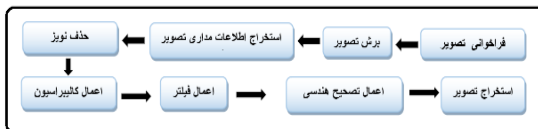
شکل ۲. مراحل پیش پردازش تصاویر ستینل-۱
