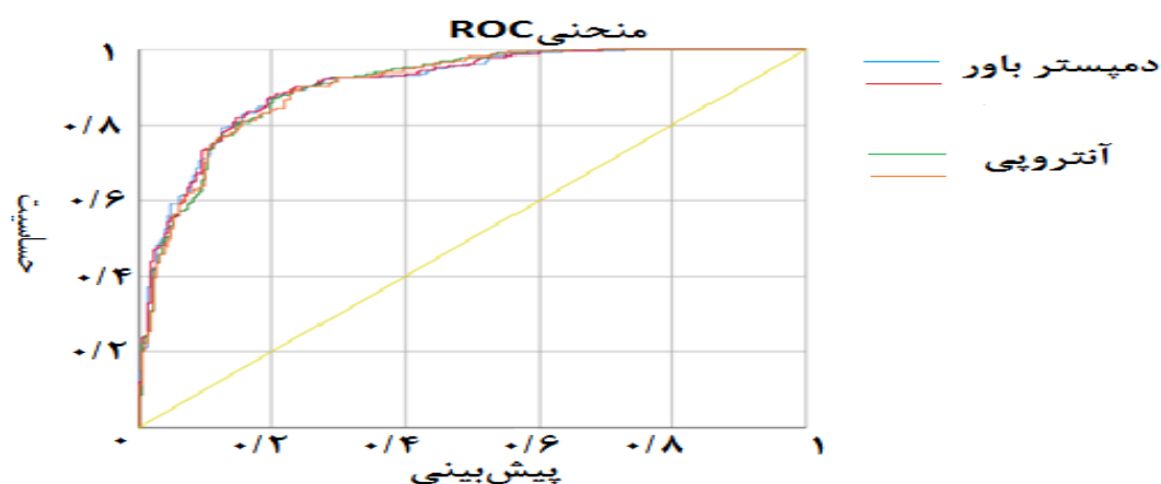
شکل ۹ نمودار منحنی مشخصه عملکرد دو مدل حداکثر آنتروپی و دمپستر-شفر در مرحله واسنجی با استفاده از ۷۰٪ پراکنش رخداد گالی‌ها
