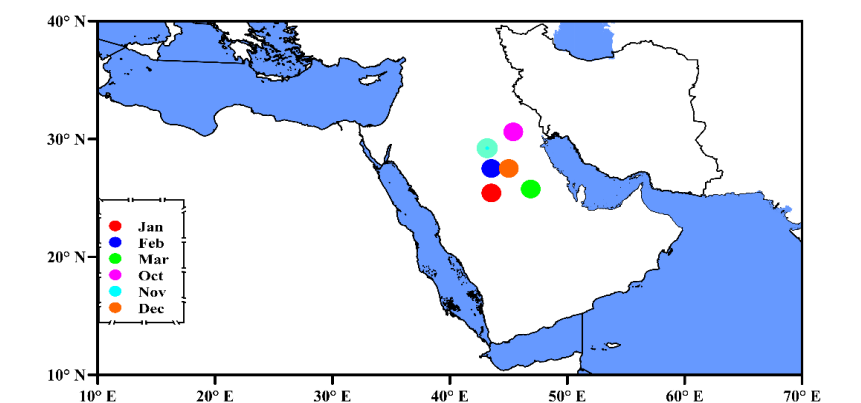
شکل ۸. موقعیت مراکز پشته پراتفیع عربستان در زمان خشکسالی ایران برای ماه‌های سرد سال
