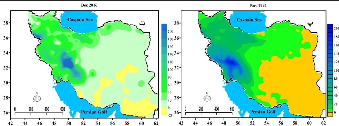
شکل ۱۱. ناهنجاری بارش برای دوره ۱۹۹۳، مارس ۲۰۱۹، نوامبر ۱۹۹۴ و دسامبر ۲۰۱۶
