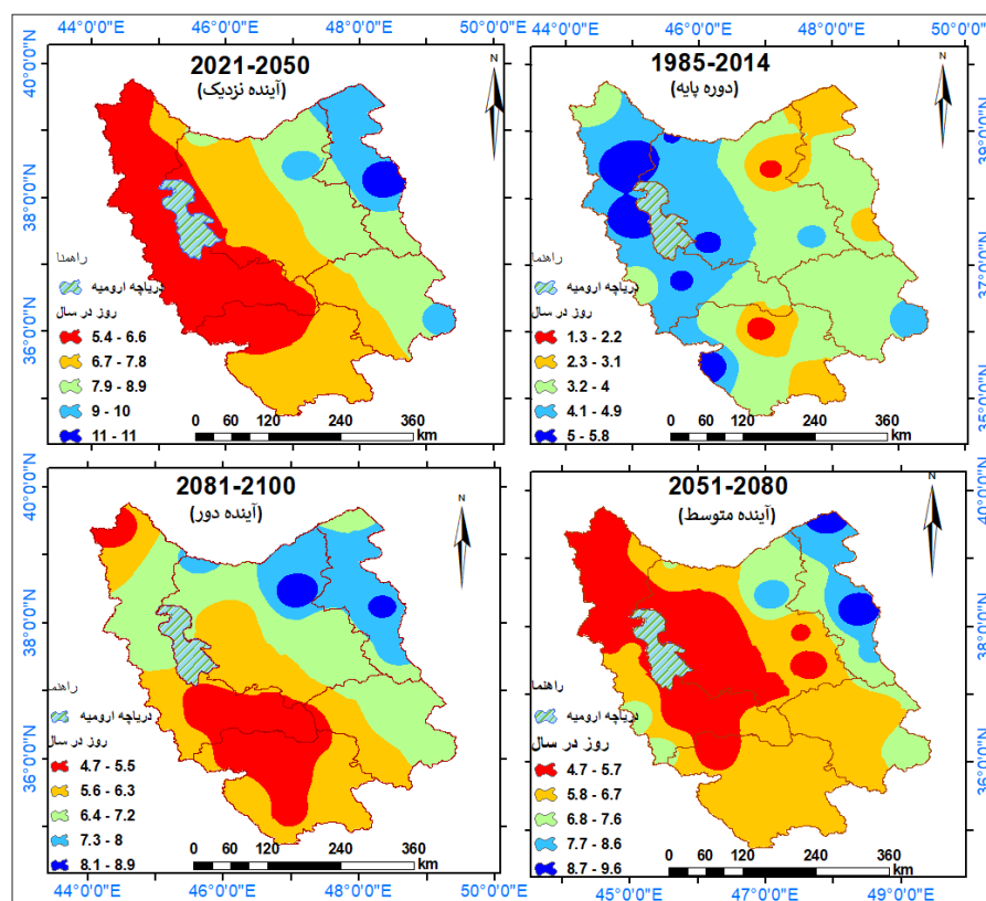
شکل ۷- توزیع فضایی شاخص CSDI با استفاده از سناریوی SSP۸.۵ در منطقه مورد بررسی
