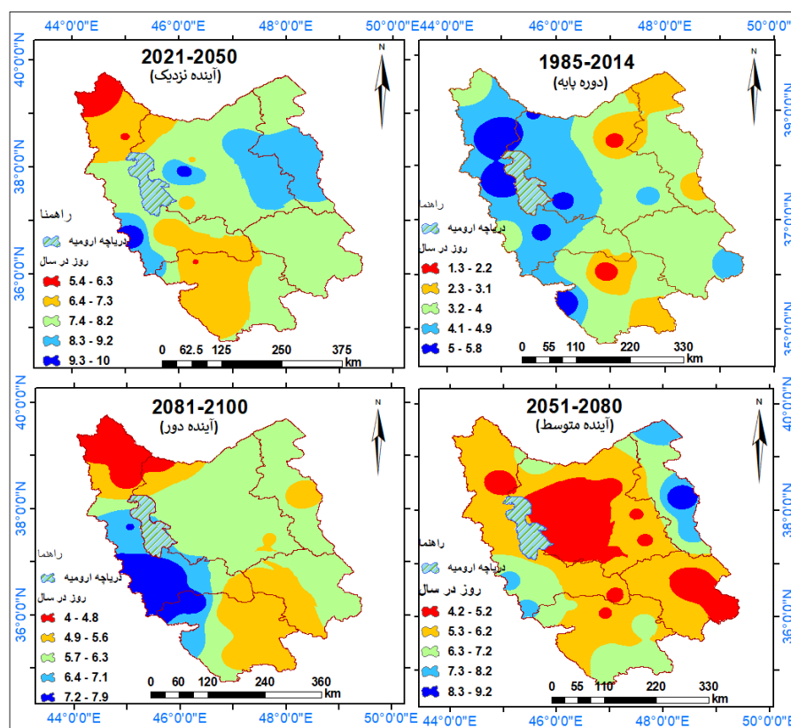
شکل ۵- توزیع فضایی نمایه CSDI با استفاده از سناریوی ۲،۶-SSP۱ در منطقه مورد بررسی
