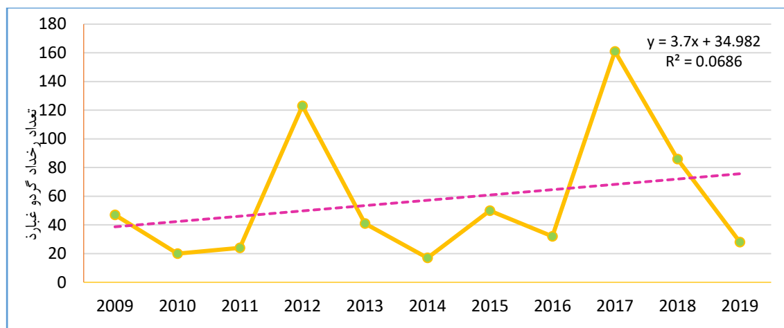
شکل ۴- فراوانی رخداد کل گرد و غبارها در ایستگاه سینوپتیک اردل
