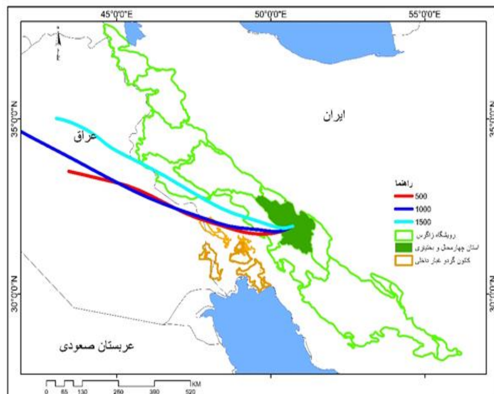
شکل ۱۱- منشأ و مسیر ورود ذرات گرد و غبار به جنگل‌های زاگرس استان چهارمحال و بختیاری از سمت شمال غرب ۰۵/۰۷/۱۳۹۹
