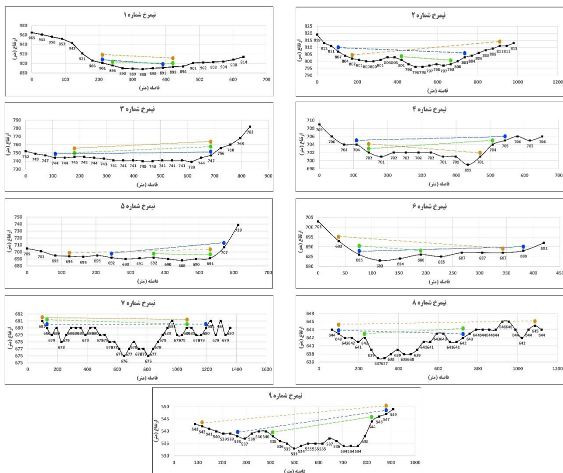
شکل ۶. نیمرخ عرضی بیجان‌رودها در محدوده مورد مطالعه. خط چین آبی متعلق به پنجم فروردین، خط چین سبز متعلق به یازدهم و خط چین قرمز متعلق به سیزدهم فروردین ۱۳۹۸ است. در نیمرخ‌ها به فاصله و ارتفاع در قسمت چپ و راست توجه شود.
