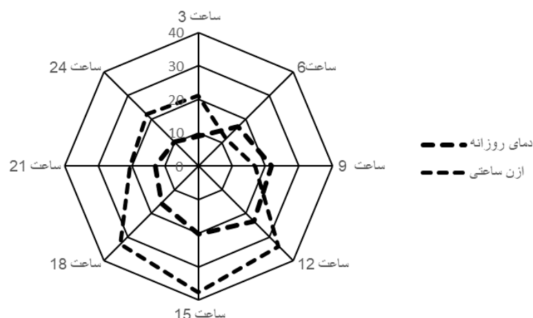
شکل ۷. نمودار تغییرات ازون ساعتی و دمای روزانه
