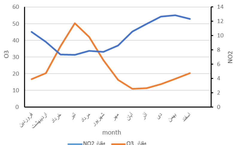
شکل ۱۸. مقدار غلظت ازون ساعتی و دی اکسید نیتروژن
