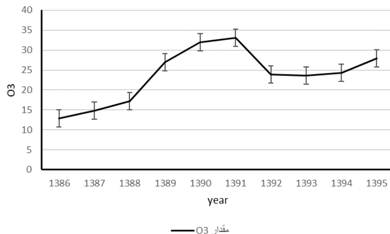
شکل ۲. مقدار اوزون سالانه
