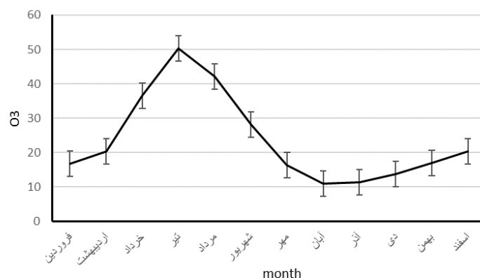
شکل ۳. مقدار اوزون ماهانه
