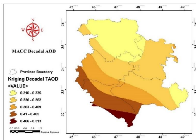
شکل (۵). نقشه توزیع مکانی میانگین سالانه AOD 550nm برای MACC در غرب ایران (۲۰۱۲-۲۰۰۳)
