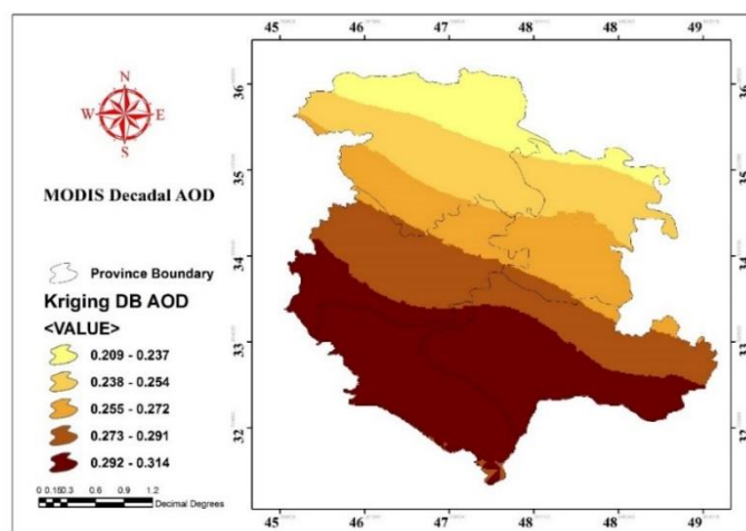
شکل (۶). نقشه توزیع مکانی میانگین سالانه AOD 550nm برای MODIS در غرب ایران (۲۰۱۲-۲۰۰۳)
