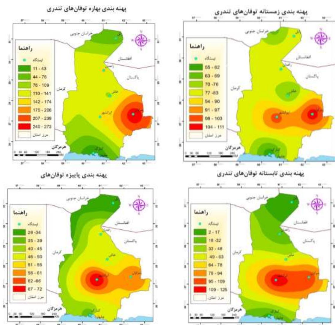
شکل ۷: پهنه بندی توفان‌های تندر در فصول مختلف سال
