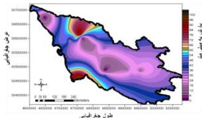
شکل ۲۶: نقشه پهنه بندی بارش سنگین در روز ۱۷ نوامبر ۱۹۹۴
