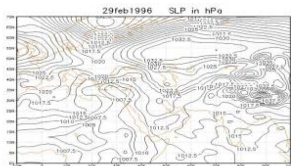
شکل ۹: نقشه آرایش الگوهای فشار سطح زمین (SLP) در روز ۲۹ فوریه ۱۹۹۶
