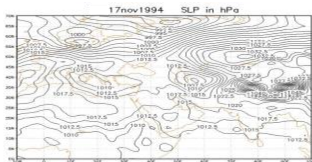
شکل ۲۱: نقشه آرایش الگوهای فشار سطحزمین (SLP) در روز ۱۷ نوامبر ۱۹۹۴
