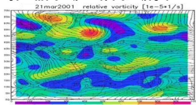
شکل ۳۰: نقشه تاوایی و خطوط جریان تراز ۱۰۰۰ هکتوپاسکال در روز ۲۱ مارس ۲۰۰۱
