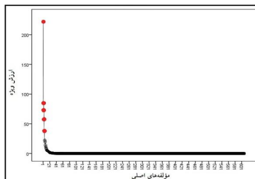
شکل (۴): نمودار پلکانی تحلیل مؤلفه‌های اصلی بر روی داده‌های تراز سطح دریا
