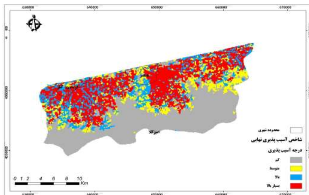
شکل ۸. نقشه نهایی آسیب پذیری سواحل شهرستان بابل برای بالا آمدن آب دریا
