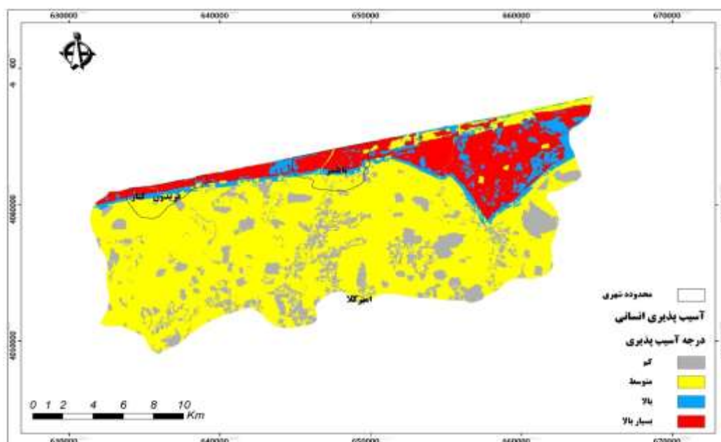
شکل ۷. نقشه آسیب پذیری سواحل شهرستان بابل بر اساس شاخص آسیب پذیری طبیعی
