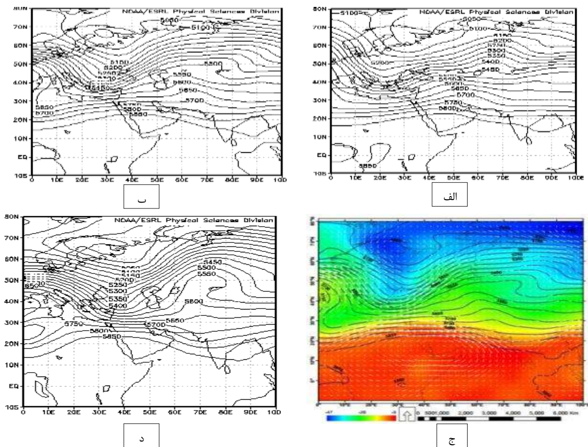
شکل ۲: نقشه‌ی الگوی فشار سطح ۵۰۰ هکتوپاسکال. (الف) روز ۱۷ ژانویه ۱۹۸۶ (روز قبل از وقوع کولاک)؛ (ب) روز ۱۸ ژانویه ۱۹۸۶ (روز رخداد کولاک)؛ (ج) نقشه‌ی ترکیبی فشار سطح ۵۰۰ با دما و باد روز ۱۸ ژانویه ۱۹۸۶ (روز رخداد کولاک)؛ (د) روز ۱۹ ژانویه ۱۹۸۶ (روز بعد از رخداد کولاک).
