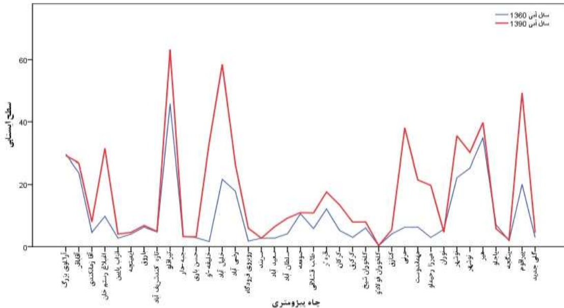
شکل ۱۳: تغییرات میانگین سطح ایستابی چاه‌های پیزومتری دشت اردبیل.
