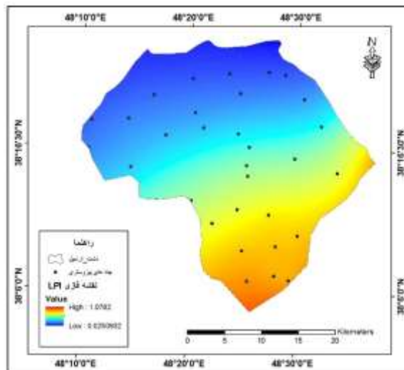
شکل ۵: نقشه فازی به روش LPI برای سال آبی ۱۳۶۰.
