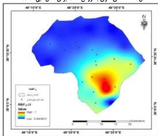
شکل ۱۰: نقشه فازی به روش RBF برای سال آبی ۱۳۹۰.
