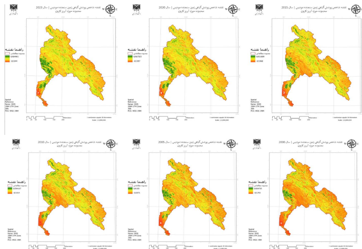
شکل ۱۹. نقشه های شاخص پوشش گیاهی حوزه آبریز کارون، میانگین سالانه ۲۰۰۰ تا ۲۰۲۳
