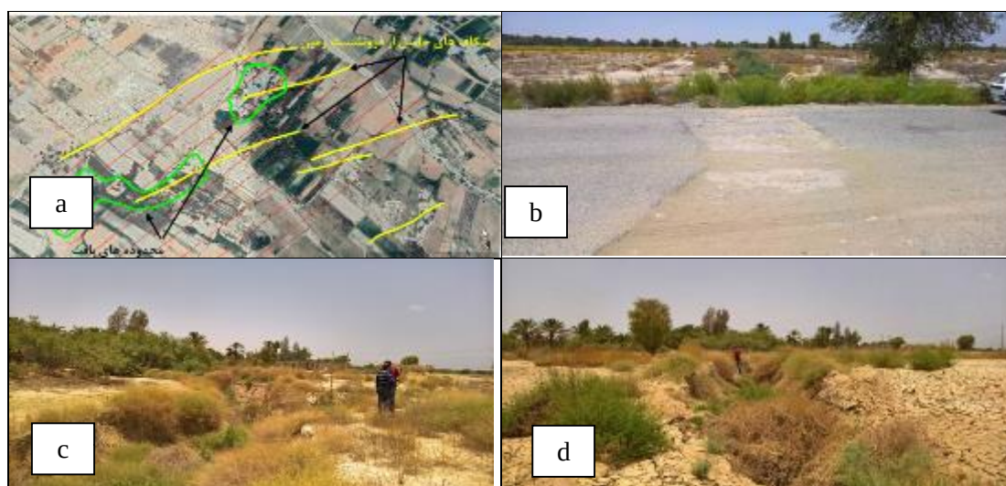
شکل ۱۰: a: موقعیت شکاف های ناشی از فرونشست زمین در اطراف روستای دول آباد، b، c و d: شکاف های ناشی از فرونشست زمین و آسیب به منازل در روستای دوآباد، e: موقعیت شکاف های ایجاد شده در روستای کهورنانجک (خطوط زرد) و محدوده های در معرض آسیب بافت مسکونی (هاشور قرمز) f، g و h: موقعیت شکاف های ناشی از فرونشست زمین در روستای کهورنانجک، i: موقعیت شکاف های ایجاد شده در محدوده پیرامونی بافت مسکونی روستای دره شور (خطوط زرد) و محدوده های در معرض آسیب بافت مسکونی (هاشور قرمز)، j: تصویری از شکاف ناشی از فرونشست زمین در روستای دره شور
