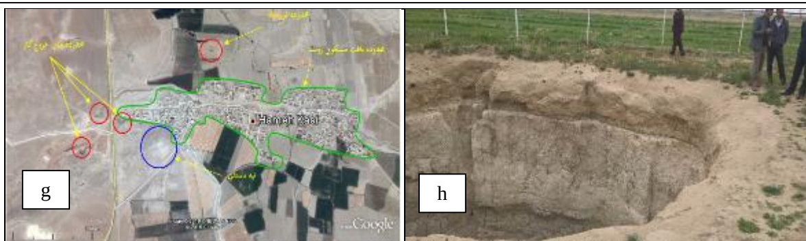
شکل ۱۴: a: نمایی از وضعیت نشست ساختمان ها در شهر فراغی b: نمایی از ترک خوردگی دیوار در اثر فرونشست در شهر فراغی، c و d: شکاف های ایجاد شده در اثر فرونشست زمین در روستای خلج، e: شکاف های ایجاد شده در اثر فرونشست زمین در روستای قادرآباد، f: بیرون زدگی لوله جدار چاه در اثر فرونشست زمین در روستای قادرآباد، g: موقعیت فروچاله نسبت به بافت مسکونی روستای همه کسی، h: فروچاله ایجاد شده در زمین های کشاورزی در ۱۵۰ متری شمال روستای همه کسی
