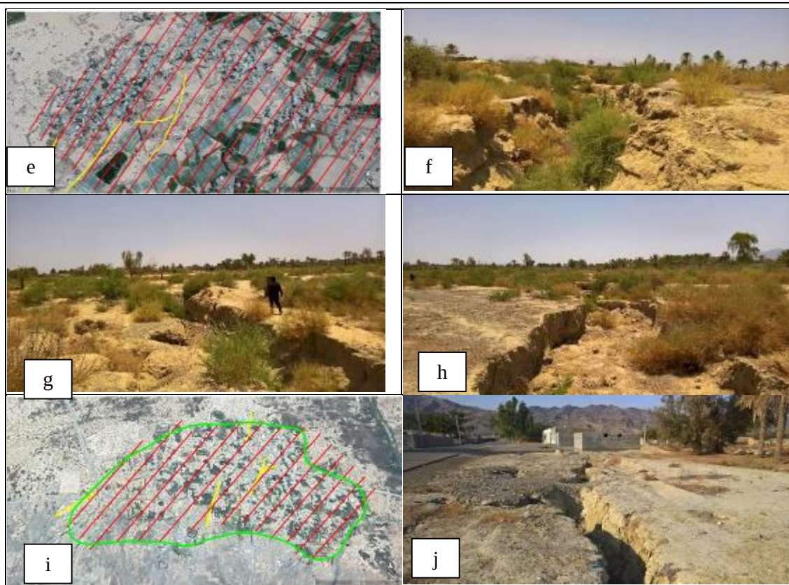
شکل ۱۰: a: موقعیت شکاف های ناشی از فرونشست زمین در اطراف روستای دول آباد، b، c و d: شکاف های ناشی از فرونشست زمین و آسیب به منازل در روستای دوآباد، e: موقعیت شکاف های ایجاد شده در روستای کهورنانجک (خطوط زرد) و محدوده های در معرض آسیب بافت مسکونی (هاشور قرمز) f، g و h: موقعیت شکاف های ناشی از فرونشست زمین در روستای کهورنانجک، i: موقعیت شکاف های ایجاد شده در محدوده پیرامونی بافت مسکونی روستای دره شور (خطوط زرد) و محدوده های در معرض آسیب بافت مسکونی (هاشور قرمز)، j: تصویری از شکاف ناشی از فرونشست زمین در روستای دره شور
