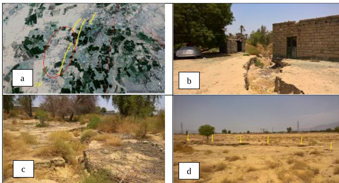
شکل ۹: a, b, c و d: شکاف ها و فروچاله ناشی از فرونشست زمین در روستای یزدل، e, f: موقعیت منازل آسیب دیده و شکاف ها و فروچاله ناشی از فرونشست زمین در روستای فاویان، g و h: ترک خوردگی ساختمان و فروچاله ناشی از فرونشست زمین در روستای ده محمد رفیع، i: موقعیت شکاف های ناشی از فرونشست زمین در اطراف روستای سفیدمراد، j: تصویری از شکاف ناشی از فرونشست زمین در اطراف روستای سفیدمراد
